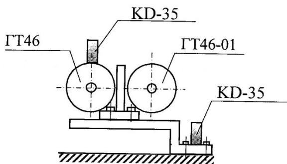
Рис. 1. Схема установки прецизионных пьезоакселерометров КД-35 при використанні кронштейна консольної конструкції
