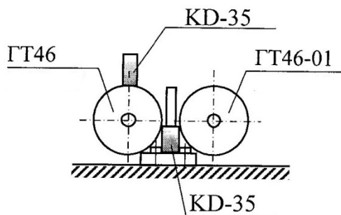
Рис. 2. Схема установки прецизионных пьезоакселерометров КД-35 при використанні кронштейна з жорстким конструктивом
