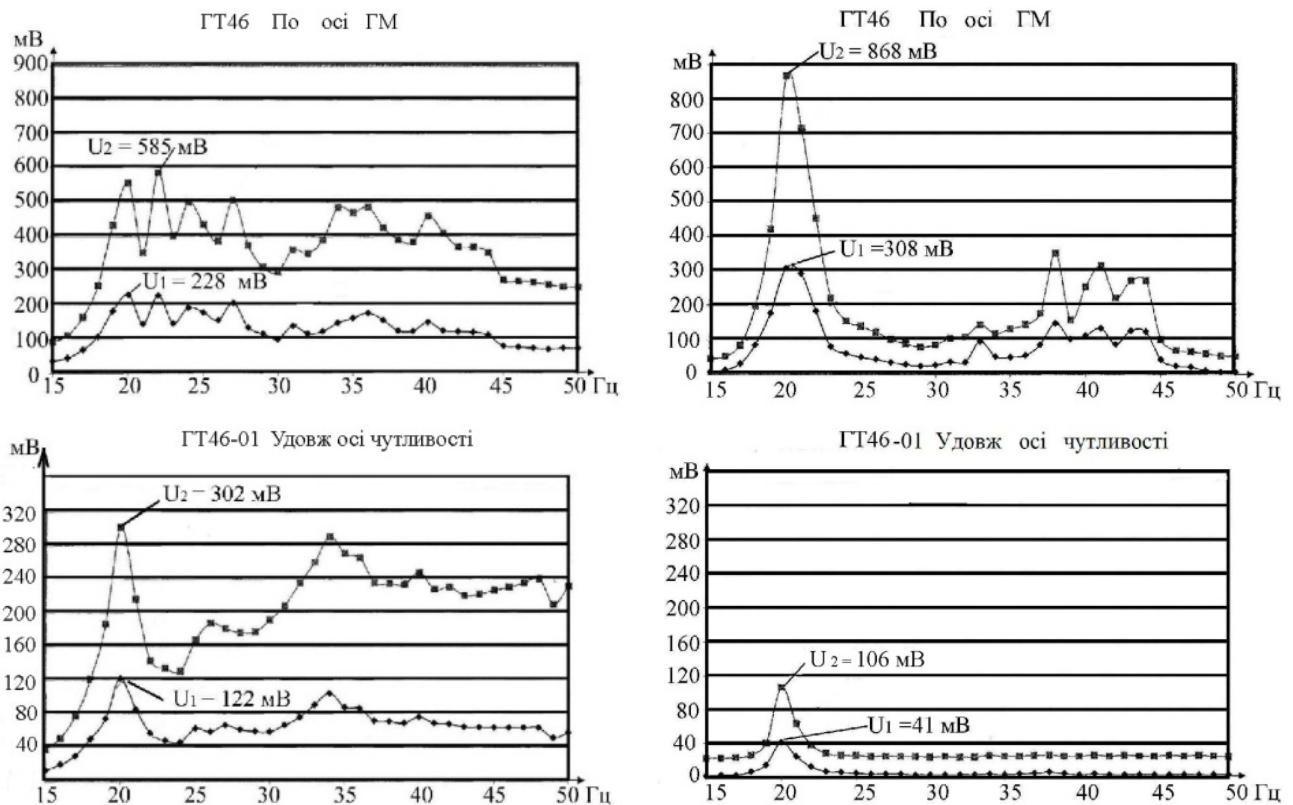
Рис. 7. Діаграми 1 випробувань консольного кріплення ГТ
