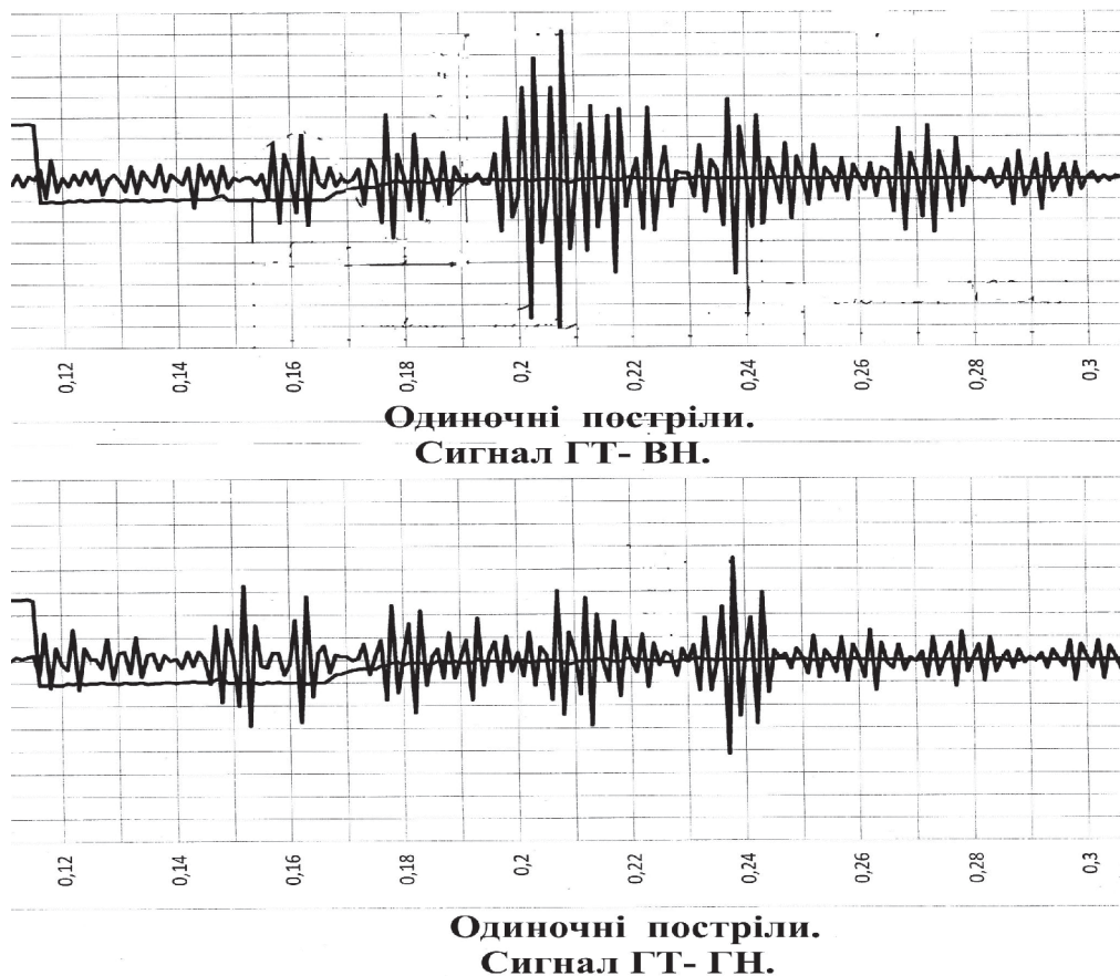
Рис. 9. Діаграми з польових випробувань консольного кріплення ГТ
