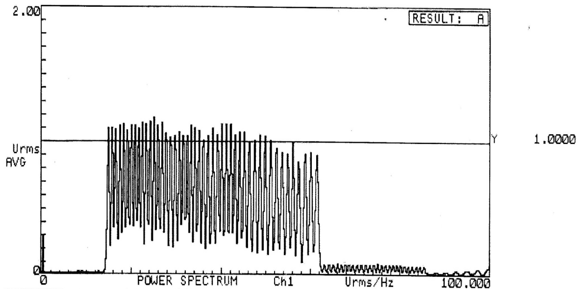
Рис. 6. Спектрограма 4
