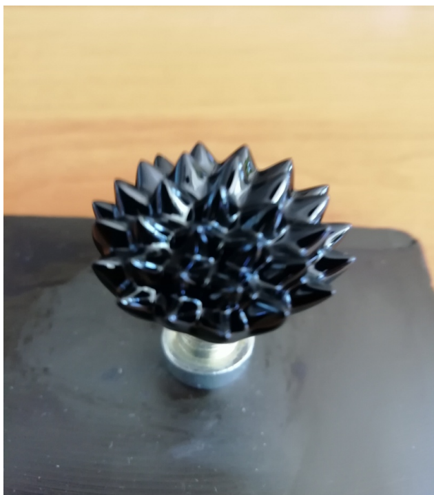
Рис. 1. Магнітна рідина
