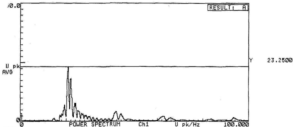
Рис. 4. Спектрограма 2
