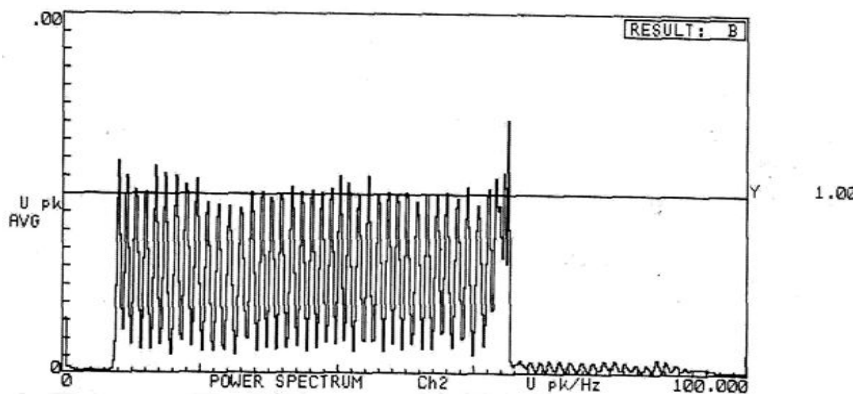
Рис. 5. Спектрограма 3
