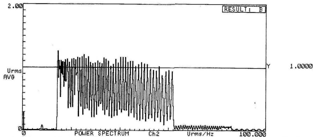
Рис. 3. Спектрограма 1
